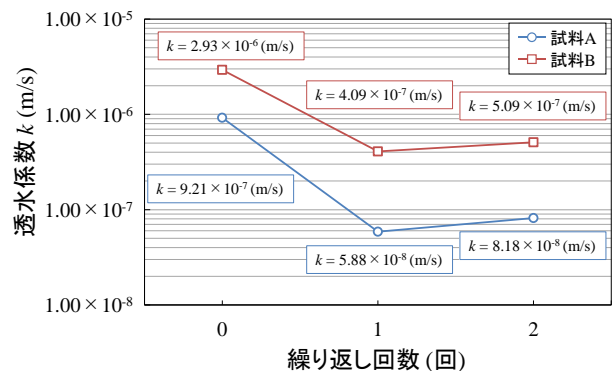
図-6 繰り返し回数ごとの透水係数
