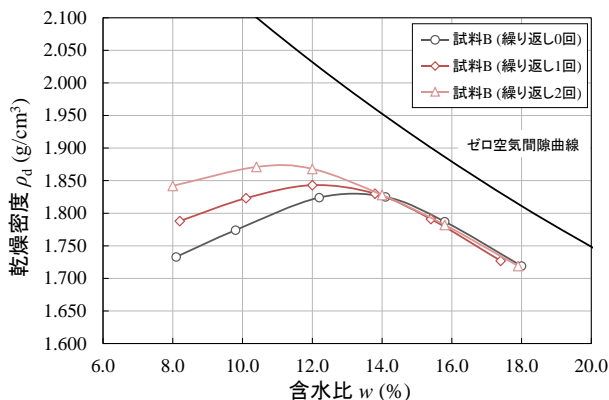
図-5 試料 B の締固め試験結果
