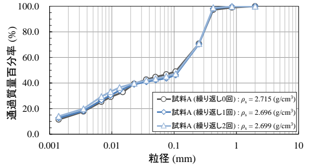
図-2 試料 A の粒径加積曲線
