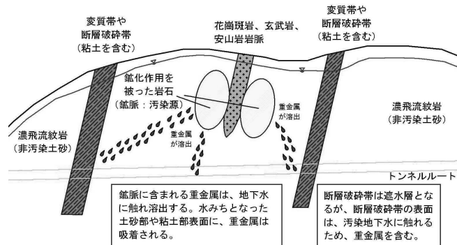
図-2 汚染土砂の出現モデル2（吸着モデル）
