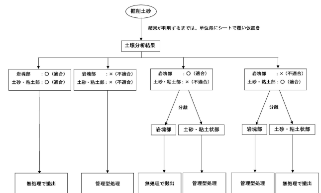
図-5 残土処理のフローチャート
