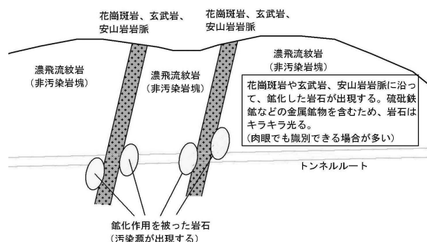
図-1 汚染土砂の出現モデル1（鉱化作用モデル）
