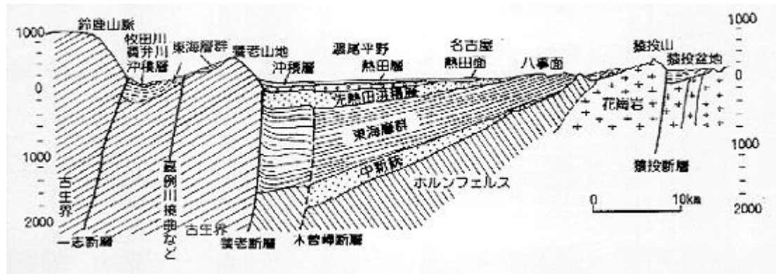
図-3 濃尾傾動地塊と周辺の東西地形・地質断面(桑原原図に岡田が加筆)
